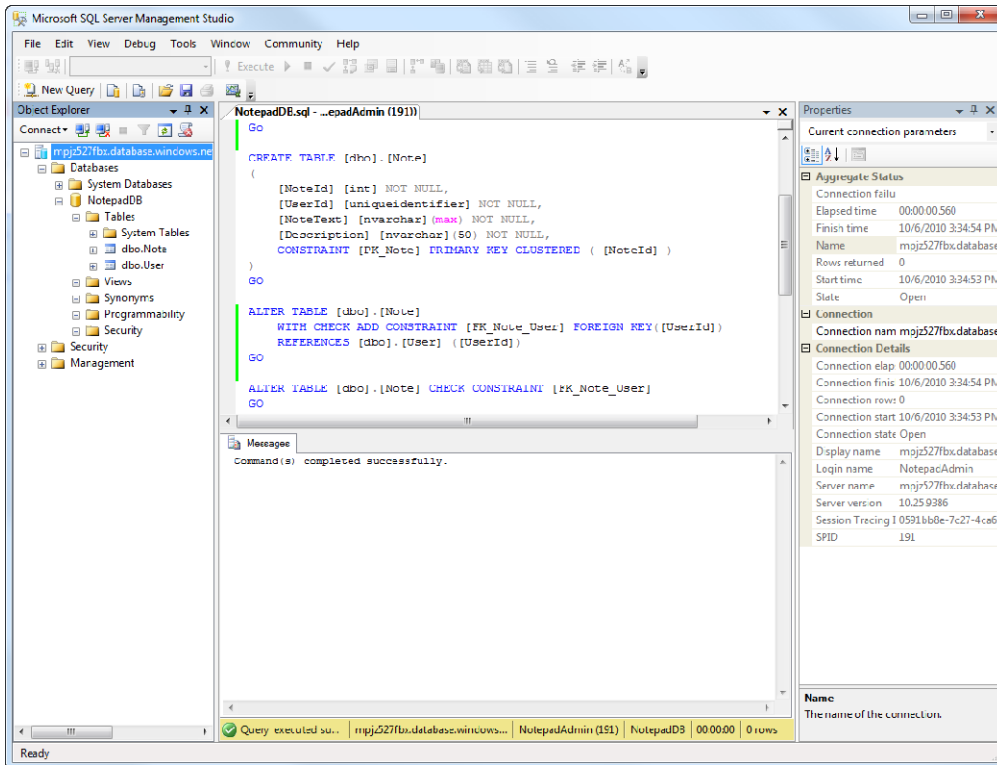
Figure 3–16. NotepadDB tables
